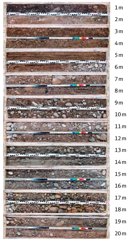
Bohrproben aus verschiedenen Tiefen (Beispielfoto)
